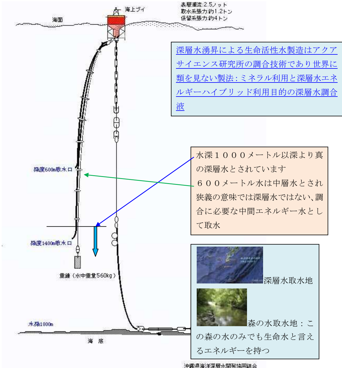
洋上設置型海洋深層水取水試験装置「海ヤカラ1号」イメージ図
